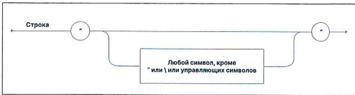
Рис. 9.4. Схема синтаксиса строки
